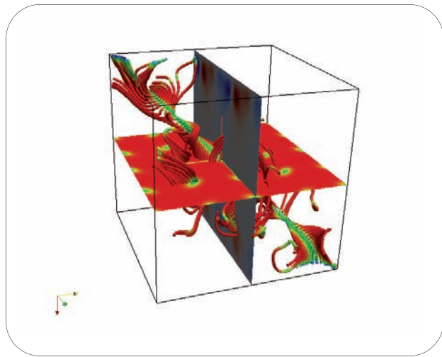
Fig. 2 Simulazione di cristalli liquidi: le sezioni orizzontale e verticale riportano zone di livello del parametro di ordine e di una componente di velocità, rispettivamente. Le linee di corrente illustrano la struttura vorticoso del campo di velocità.
