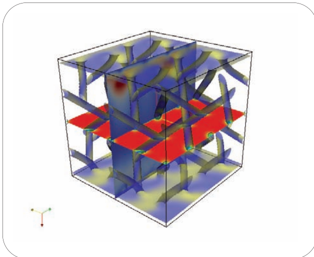
Fig. 1 Simulazione di cristalli liquidi: la struttura è visibile tramite isosuperfici e zone di livello in una sezione orizzontale del parametro di ordine. Una sezione verticale illustra il campo fluidodinamico tramite la visualizzazione di zone di livello relative al modulo del campo di velocità.
